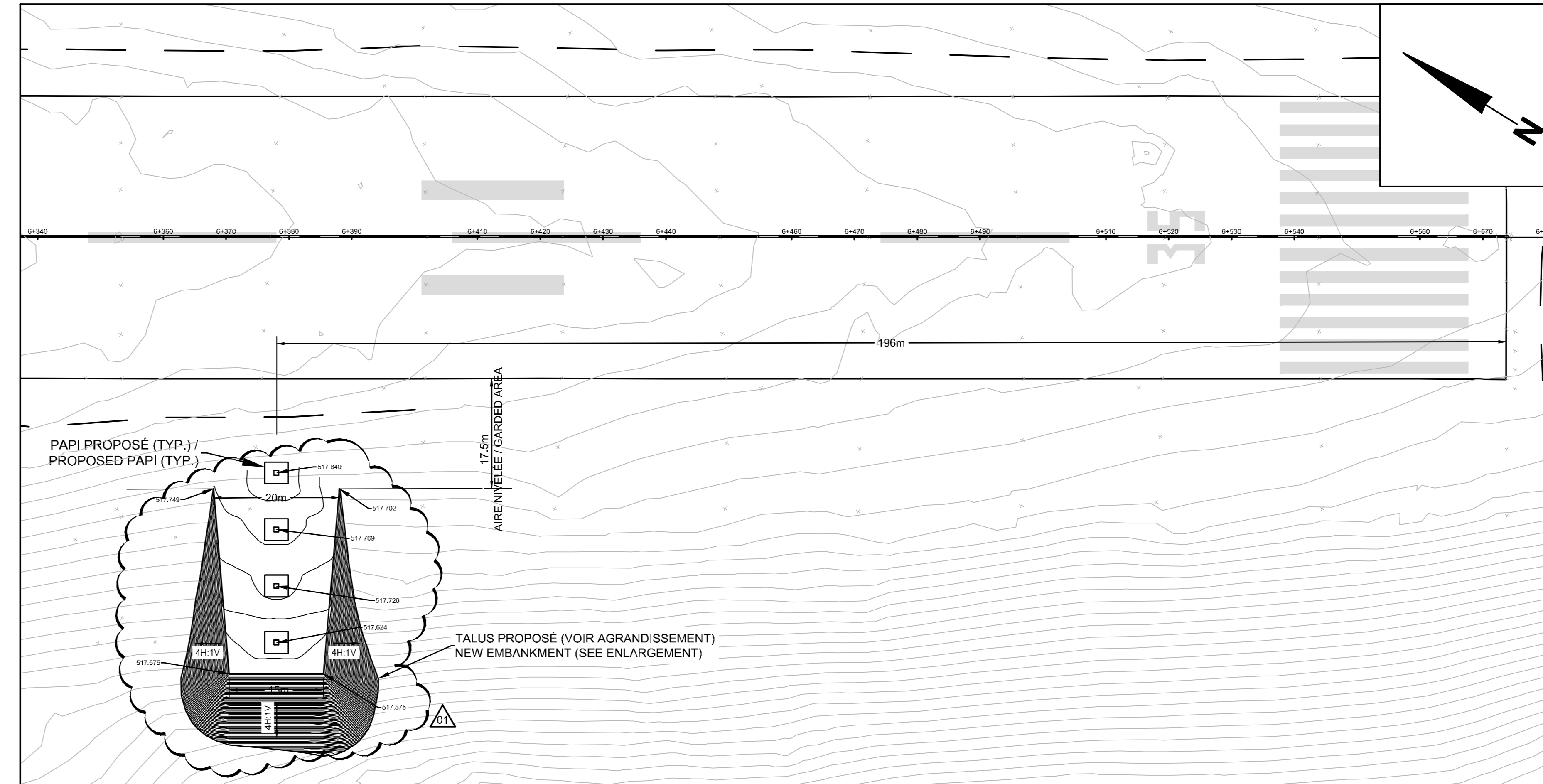
LOCALISATION DES PAPI PROPOSÉS LOCATION OF PROPOSED PAPI Echelle: 1:500
