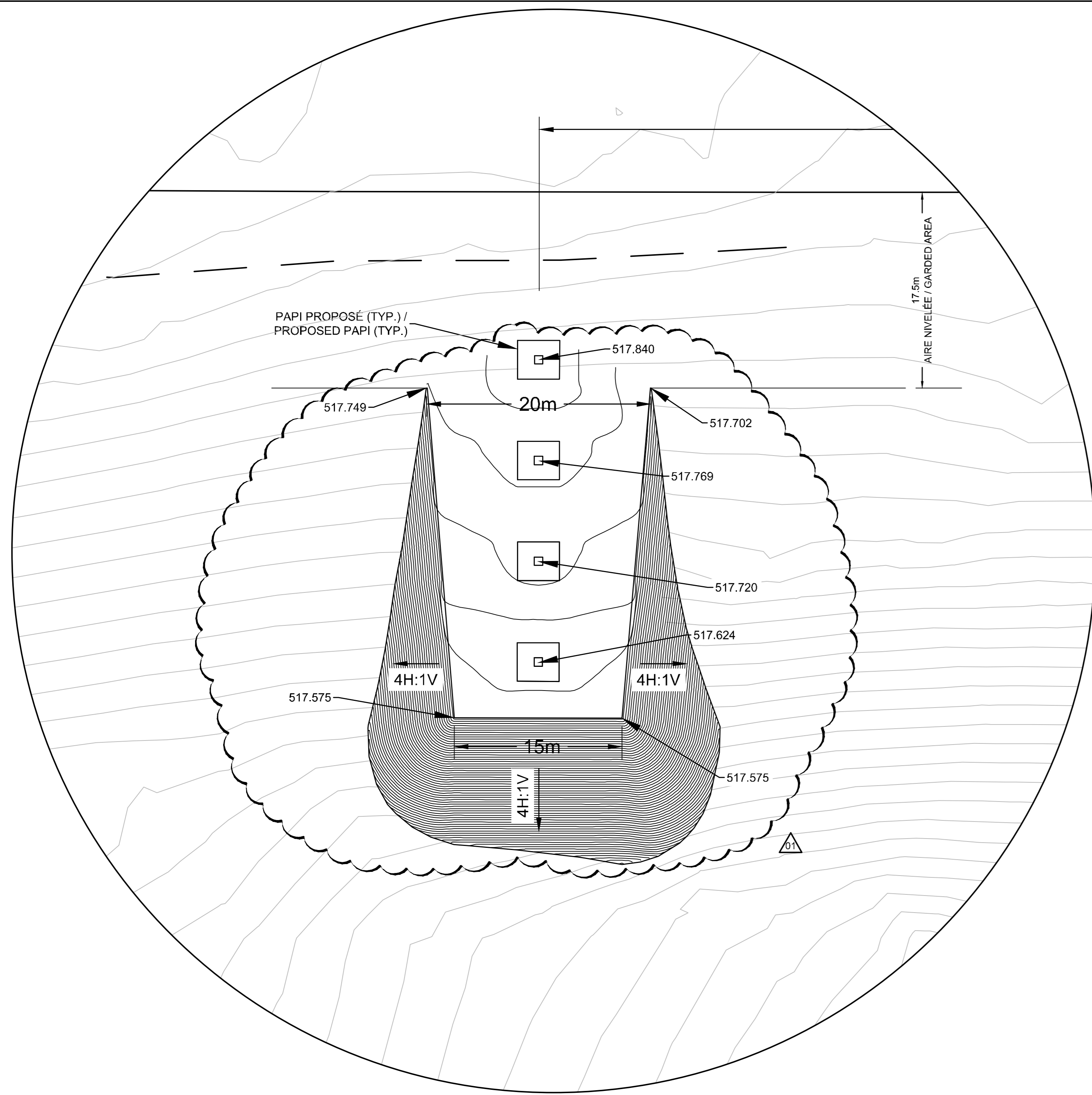
AGRANDISSEMENT DE LA VUE DU TALUS PROPOSÉ ENLARGEMENT VIEW OF THE NEW EMBANKMENT Echelle: 1:250
